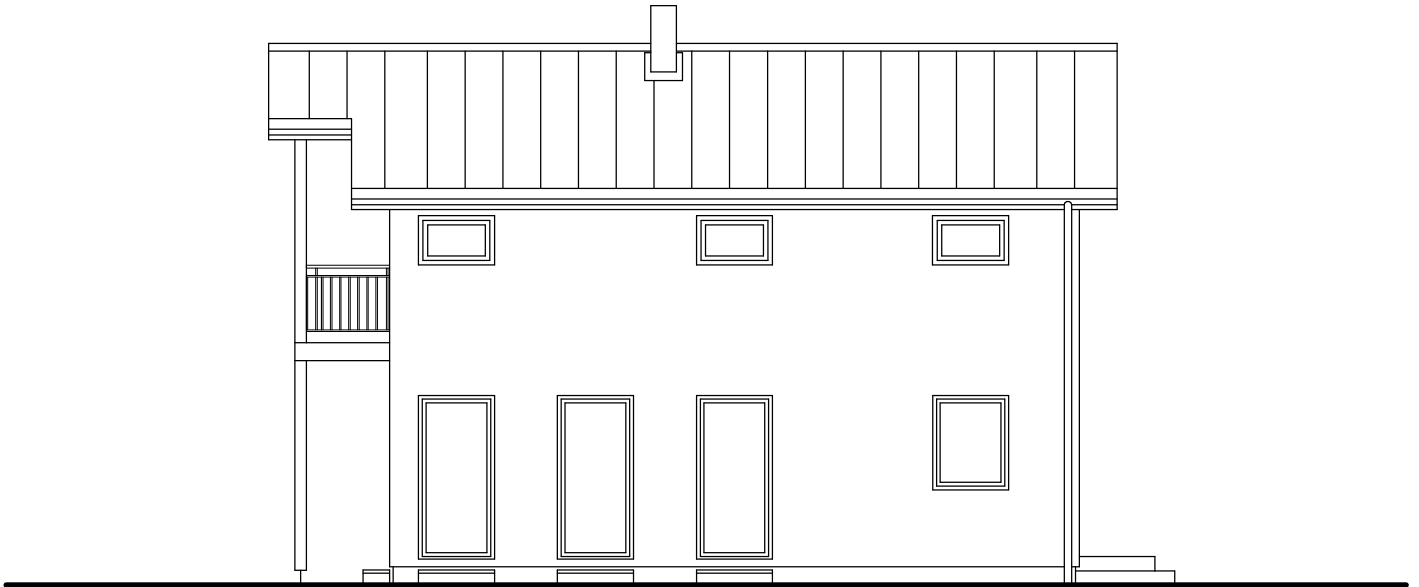
ANSICHT 1
