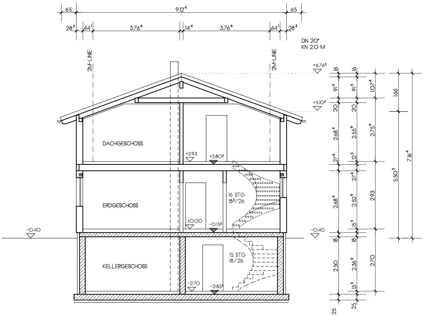
SCHNITT A-A
